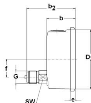
Conexión dorsal excéntrica (100mm)
