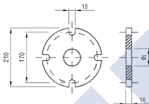
Tipo 090480 – Diámetro interior p/soldar
